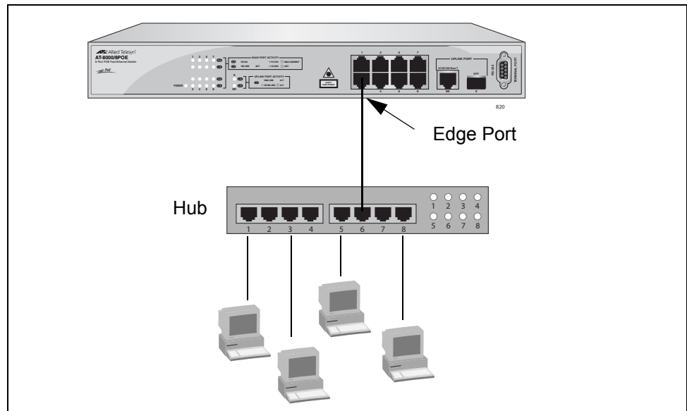
Figure 31. Edge Port
